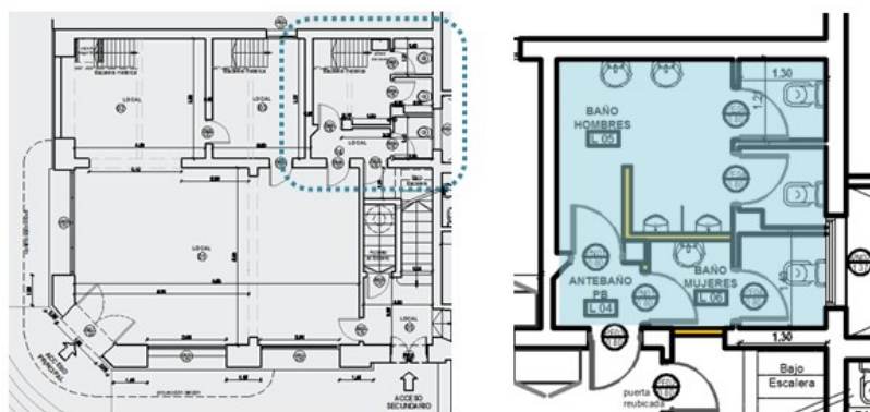
PLANTA BAJA. NUEVO NÚCLEO SANITARIO.
